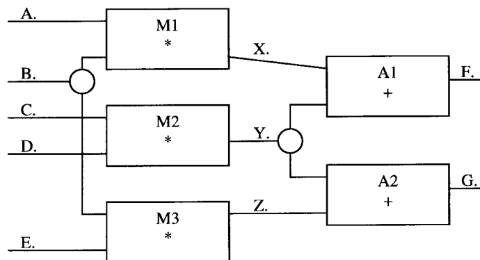
Figure 1: elektronische schakeling
