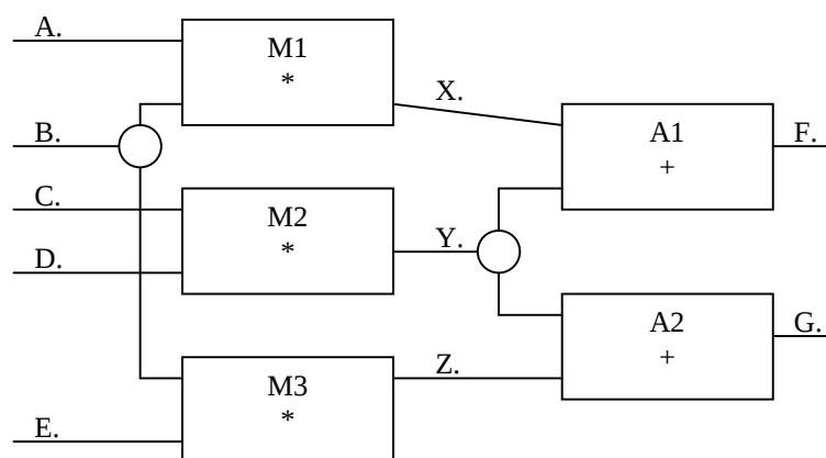
Figure 1: elektronische schakeling
