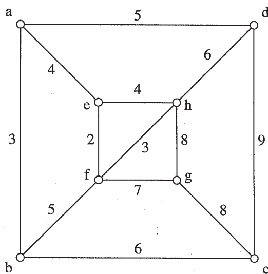
Figuur bij Opgave 1: het Prim Algoritme
