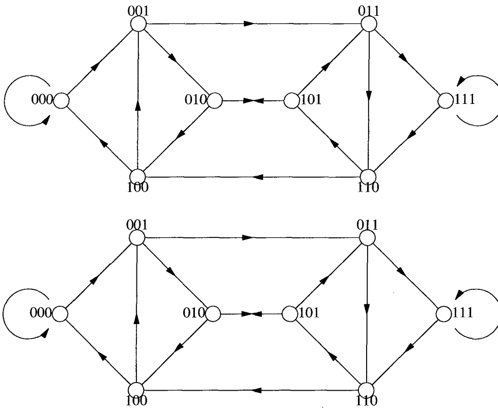
Figuur: gerichte De Bruijn graaf van orde 3
