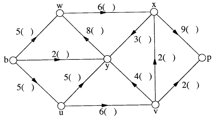
Figuur bij Opgave 1: netwerk met stroom
