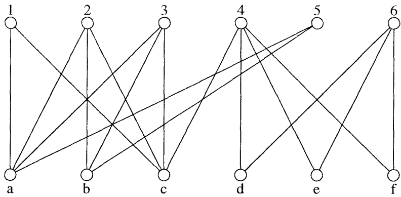
Figuur bij Opgave 3: maximum toewijzing
